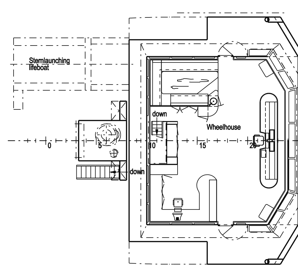
BRIDGEDECK
