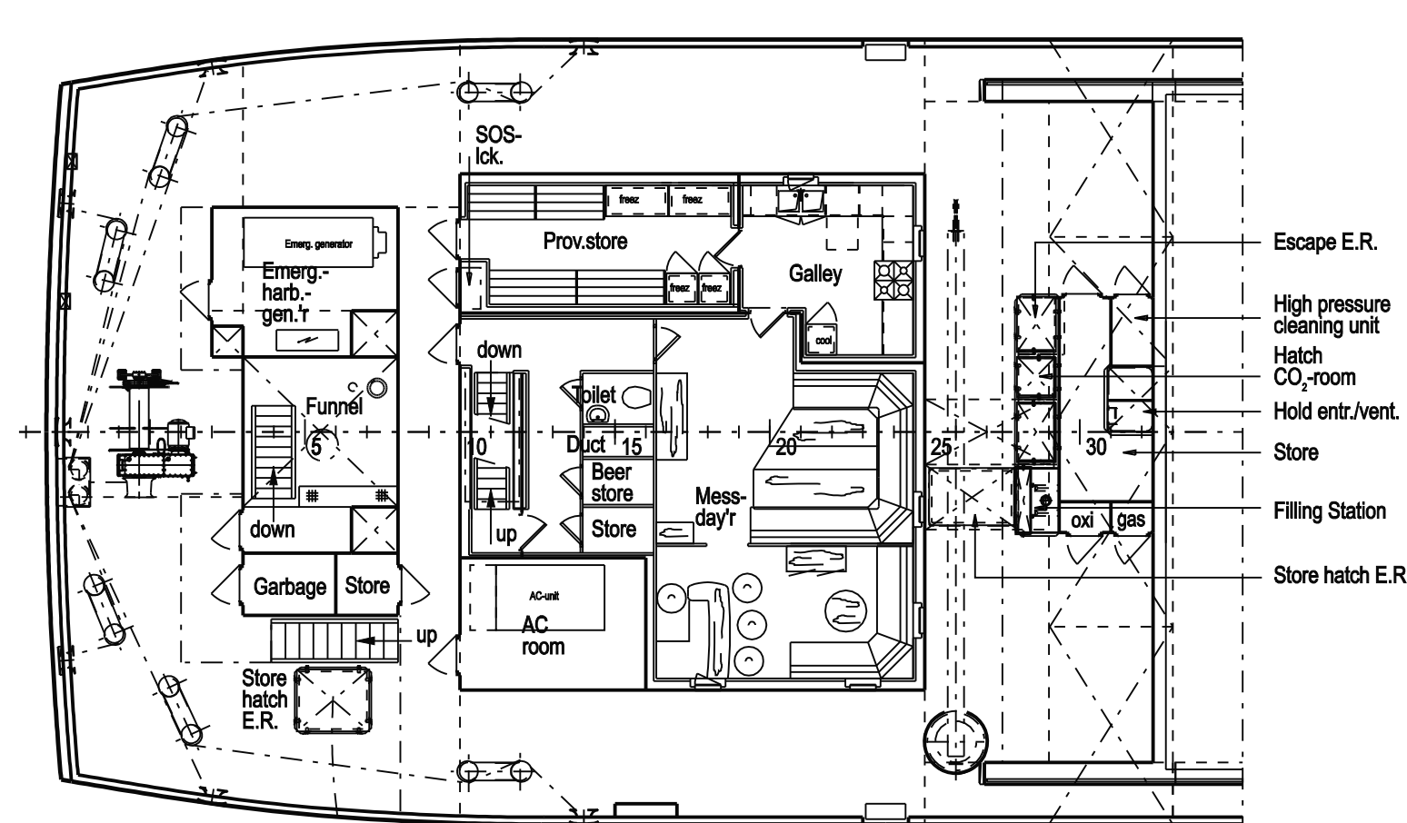
POOPDECK
